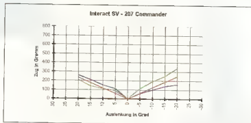
Schlecht ausgeprägte Mitte, unterschiedlicher Kraftverlauf bei den Achsen.
